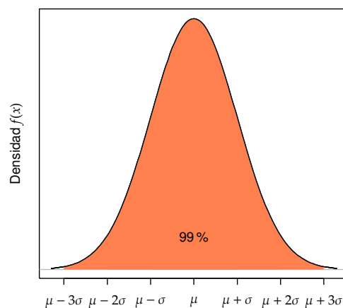
Distribución normal N(\mu, \sigma)
