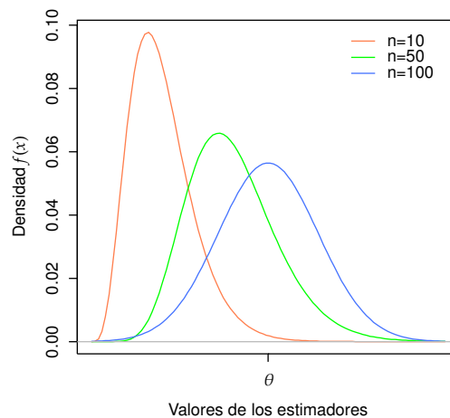
Distribuciones de estimadores asintóticamente normales
