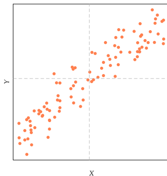
Relación lineal creciente
