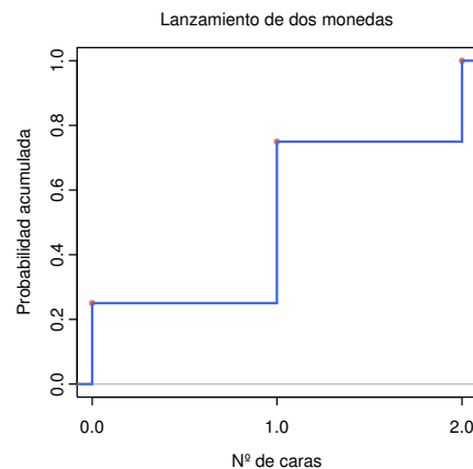
Función de distribución
