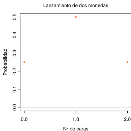
Función de probabilidad
