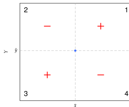
Signo del producto de desviaciones
