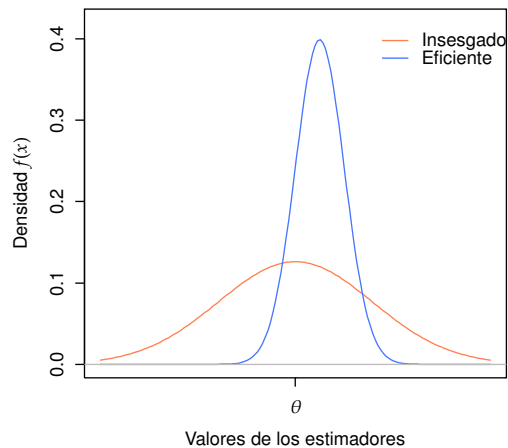
Distribuciones de estimadores incesgado y eficiente sesgado
