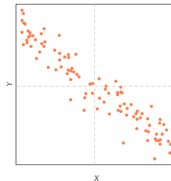
Relación lineal decreciente
